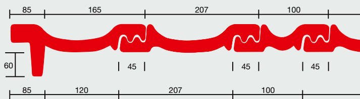
Dekkende breedte linker gevelpan 165 mm.
