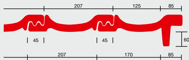
Dekkende breedte rechter gevelpan 125 mm.
